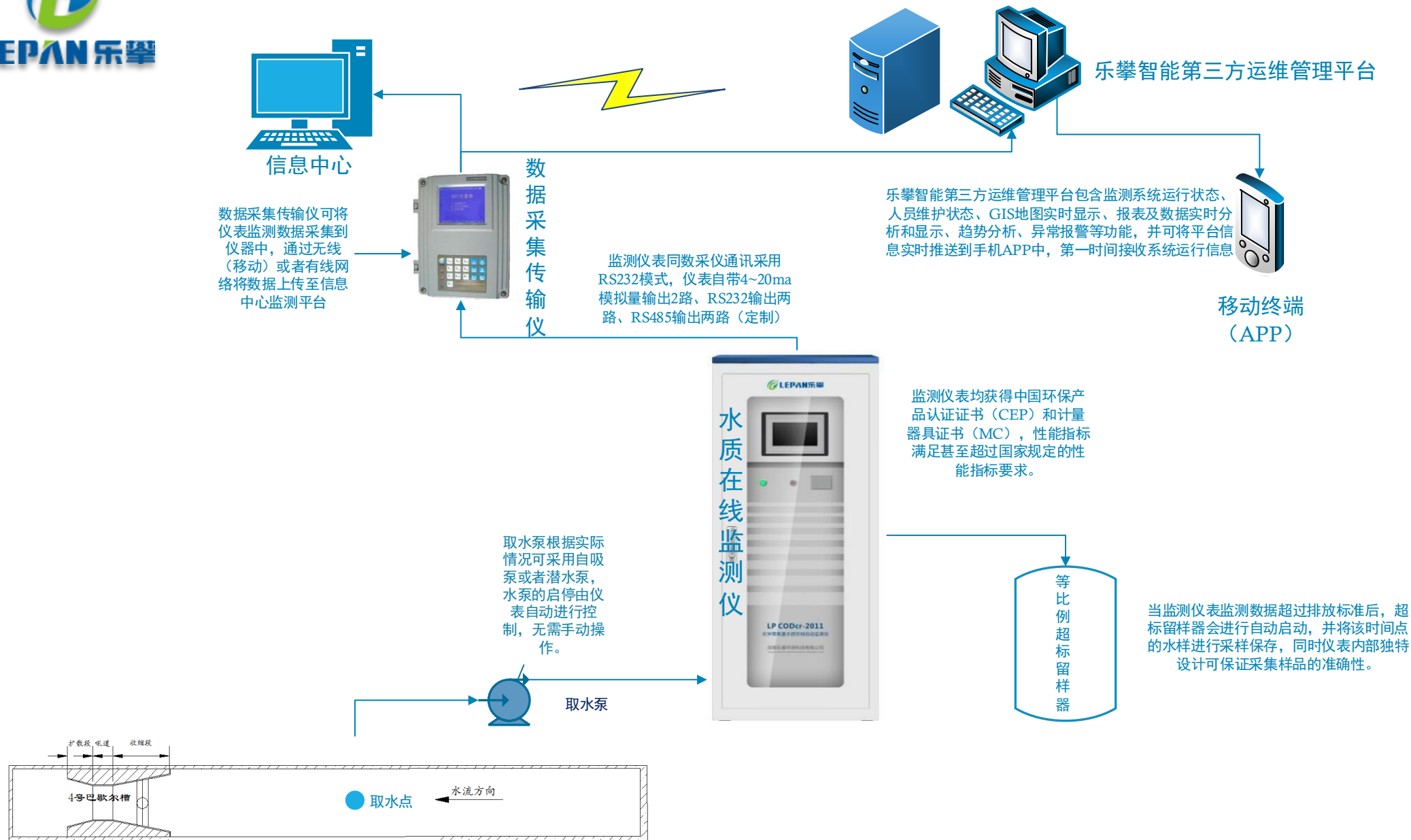
乐攀环保水质在线监测系统组织流程图
